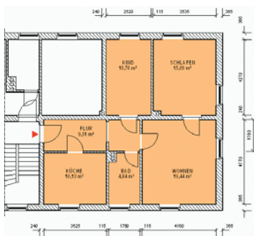
Grundriss Moderne 3-Raum-Wohnung Scharfenstein, Untere Siedlungsstraße 84,
