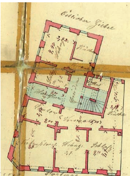
Erdgeschossgrundriss beim Neubau 1875
