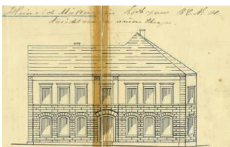
Ansicht von der Gabelsbergerstraße Bauplan 1875
