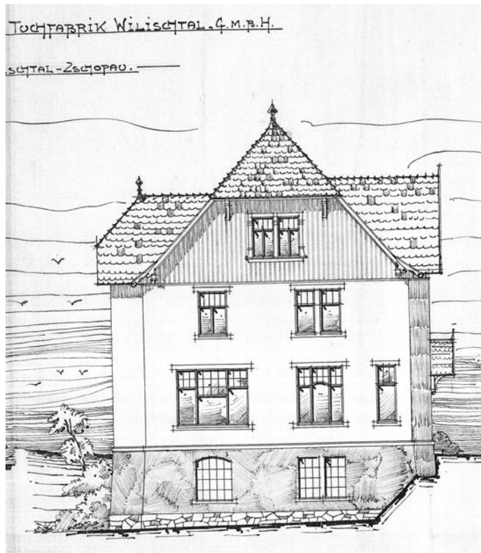
Bauzeichnung Südansicht
