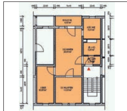
Moderne 3-Raum-Wohnung mit Balkon – 55 m² Bertolt-Brecht-Straße 7 in Zschopau
